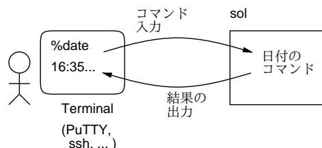
図 2.1: CUI の概念
